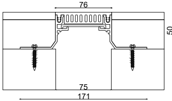
Z-1175-75W76 H50
