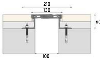
■ Z-1670A 100W130 JW :100 H:60 S:130 BW:210 M:32
