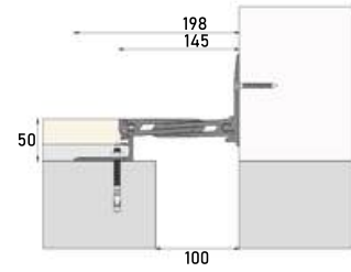
■ ZK-1670A 100W145 JW :100 H:50 S:145 BW:198 M:32
